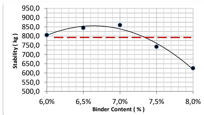
Gambar 3 Hubungan kadar aspal vs stabilitas
