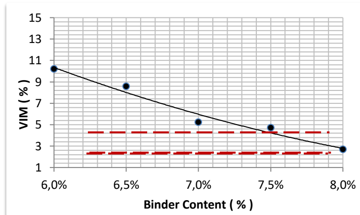
Gambar 6 Hubungan kadar aspal vs VIM
