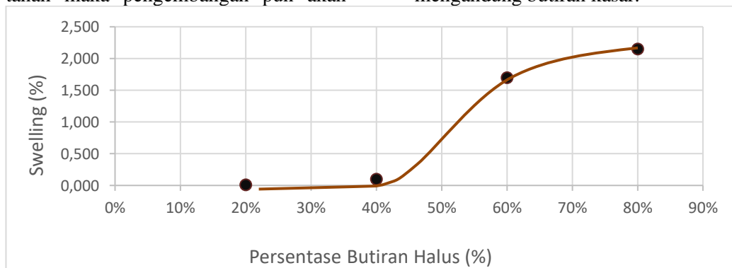
Gambar 5 Hubungan persentase butiran halus terhadap swelling
