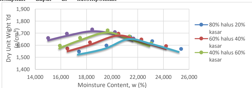
Gambar 3 Hubungan \gamma_d dan kadar air dari setiap variasi butiran tanah
