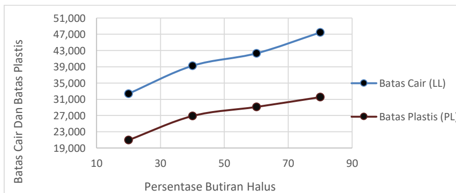
Gambar 1 Hubungan variasi butiran dengan batas cair (LL) dan batas plastis (PL)
