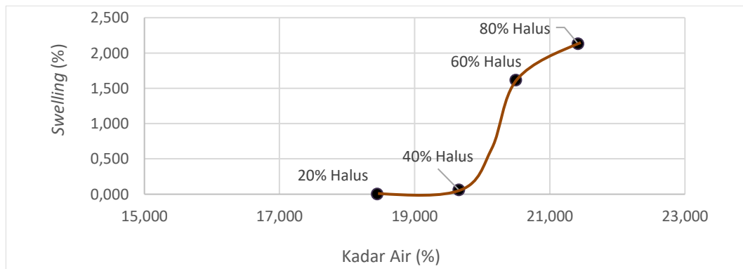
Gambar 6 Hubungan persentase butiran halusterhadap swelling
