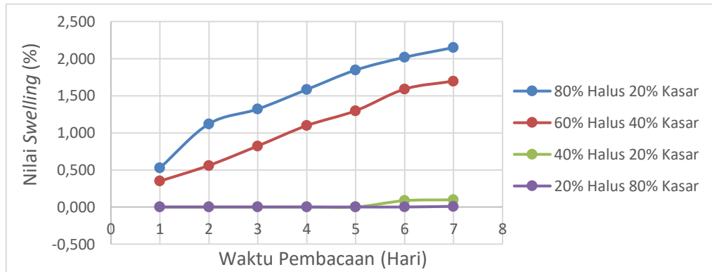
Gambar 4 Hubungan swelling dengan lama waktu perendaman setiap variasi butiran
