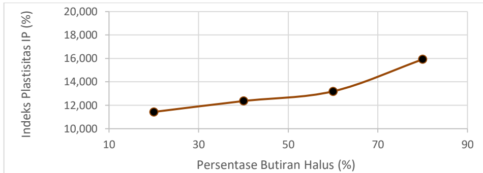
Gambar 2 Hubungan variasi butiran dengan indeks plastisitas (IP)
