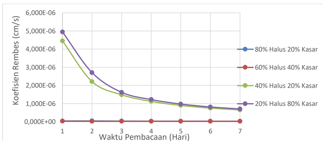
Gambar 7 Hubungan Koefisien Rembes dengan lama waktu perendaman setiap variasi butir.
